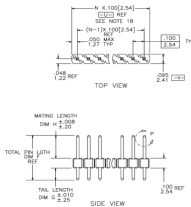
Pins dimensions
