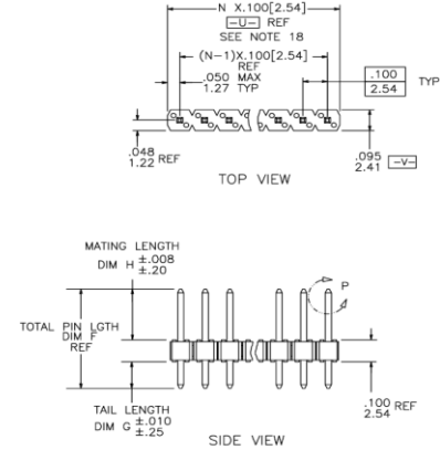
PINS DIMENSIONS
