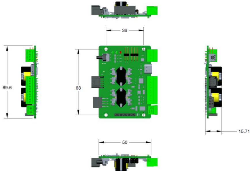
ECU Dimensions
