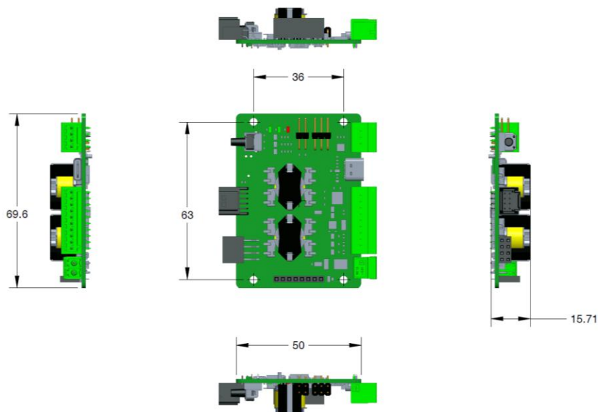
ECU Dimensions
